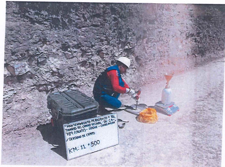
FIGURA N° 47. Ensayo de Densidad de Suelo en Campo. Progresiva 11 + 500 (Método del cono de arena).
