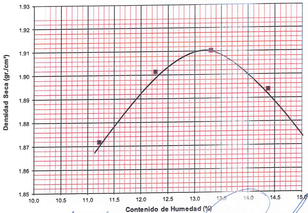
Proctor Modificado " C "
