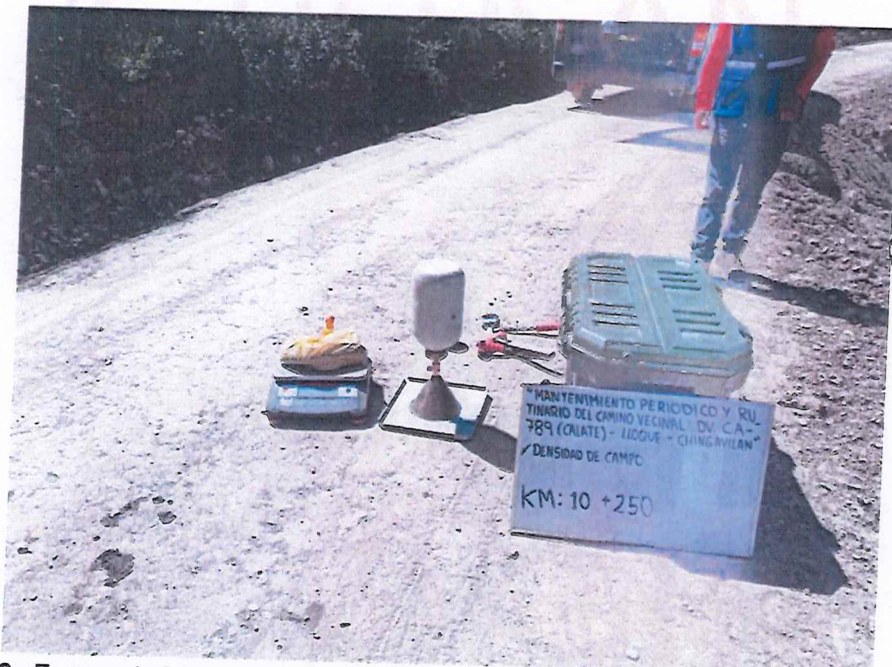
FIGURA N° 42. Ensayo de Densidad de Suelo en Campo. Progresiva 10 + 250 (Método del cono de arena).
