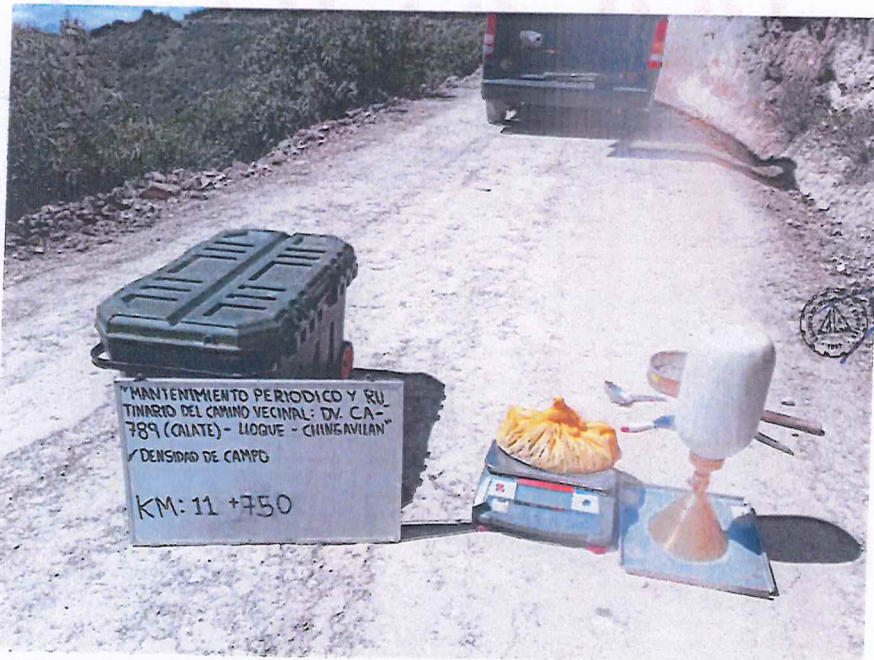
FIGURA N° 48. Ensayo de Densidad de Suelo en Campo. Progresiva 11 + 750 (Método del cono de arena).
