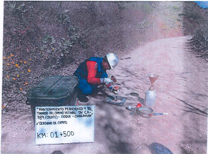
FIGURA N° 7. Ensayo de Densidad de Suelo en Campo. Progresiva 01 + 500 (Método del cono de arena).
