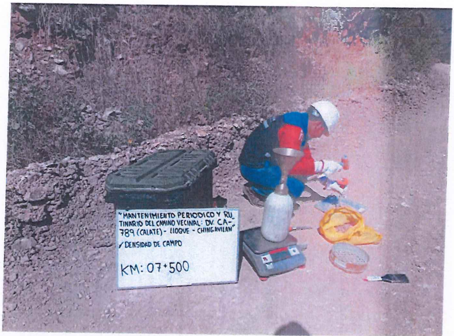
FIGURA N° 31. Ensayo de Densidad de Suelo en Campo. Progresiva 07 + 500 (Método del cono de arena).
