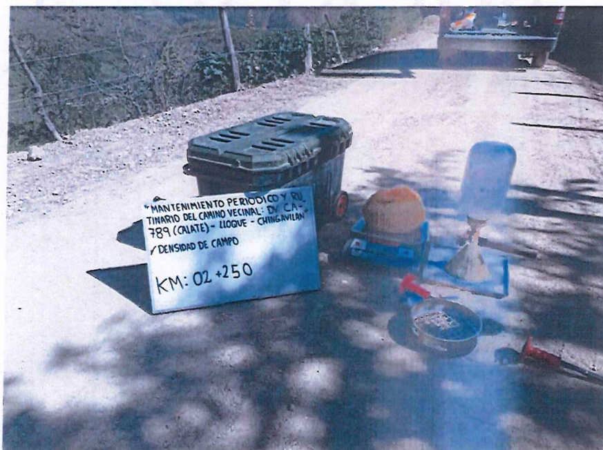
FIGURA N° 10. Ensayo de Densidad de Suelo en Campo. Progresiva 02 + 250 (Método del cono de arena).
