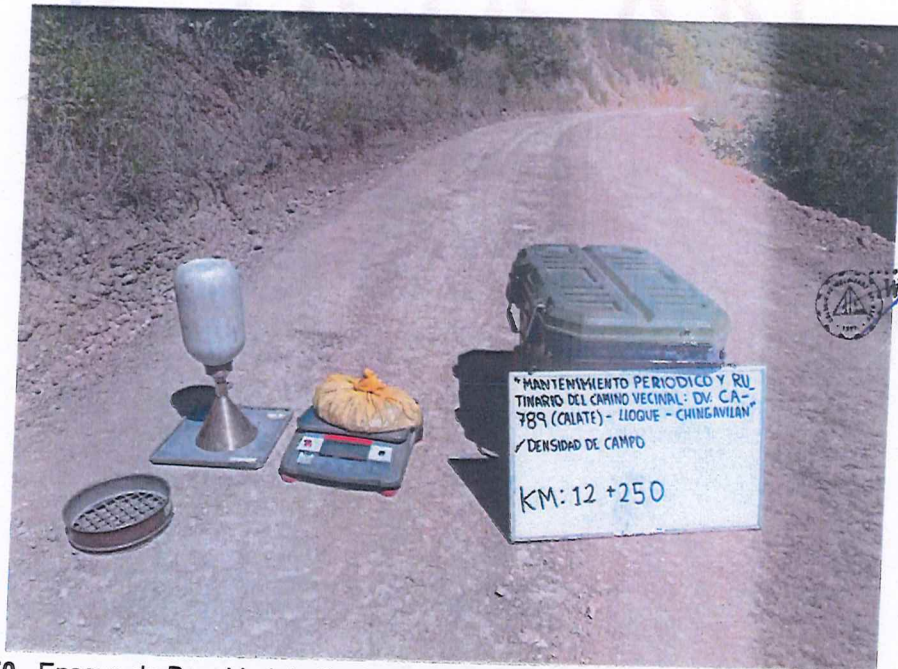
FIGURA N° 50. Ensayo de Densidad de Suelo en Campo. Progresiva 12 + 250 (Método del cono de arena).
