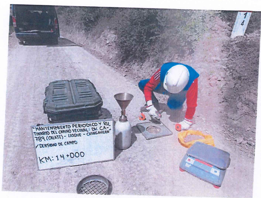
FIGURA N° 57. Ensayo de Densidad de Suelo en Campo. Progresiva 14 + 000 (Método del cono de arena).
