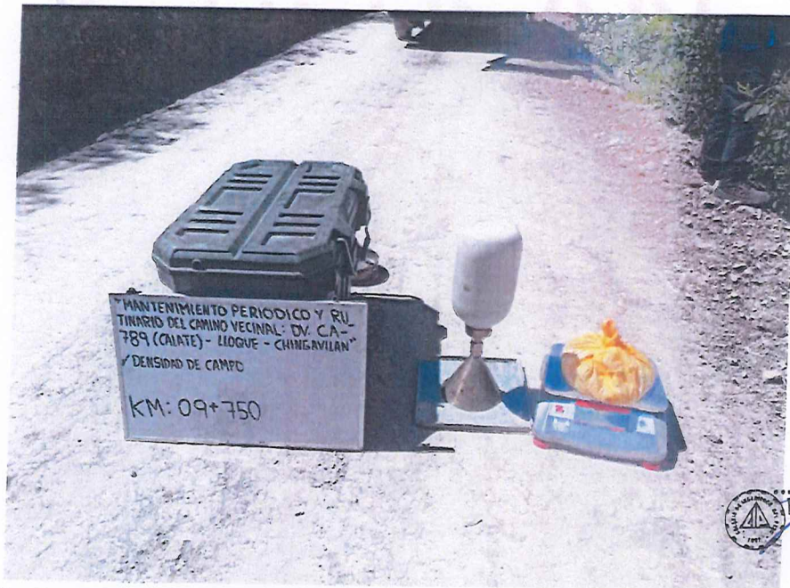
FIGURA N° 40. Ensayo de Densidad de Suelo en Campo. Progresiva 09 + 750 (Método del cono de arena).
